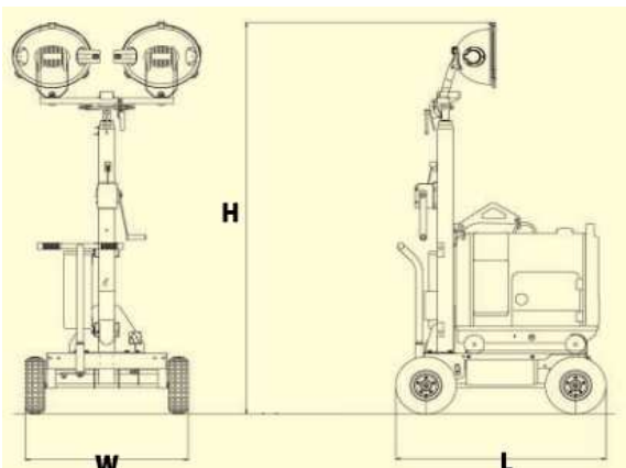
LB230 (寸法図)
